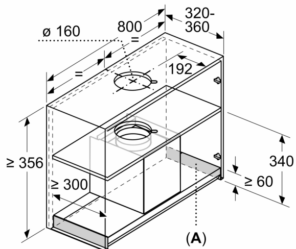
Mål i mm Indbygningseksempel
