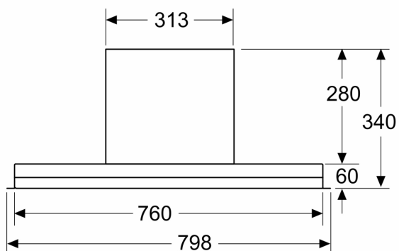
Mål i mm Set forfra
