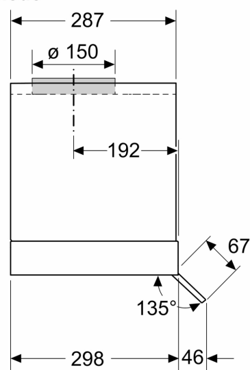
Mål i mm Sidebillede
