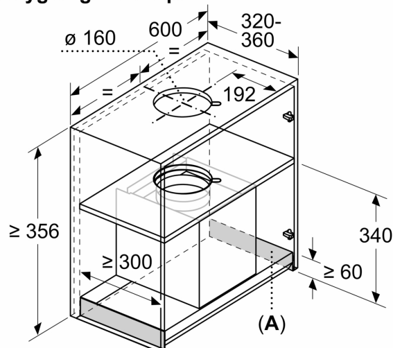
Mål i mm Indbygningseksempel
